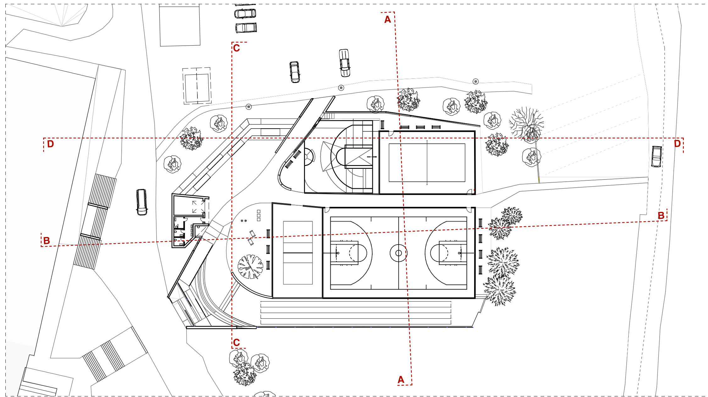
PLANIMETRIA POSIZIONE SEZIONI - SCALA 1:500
