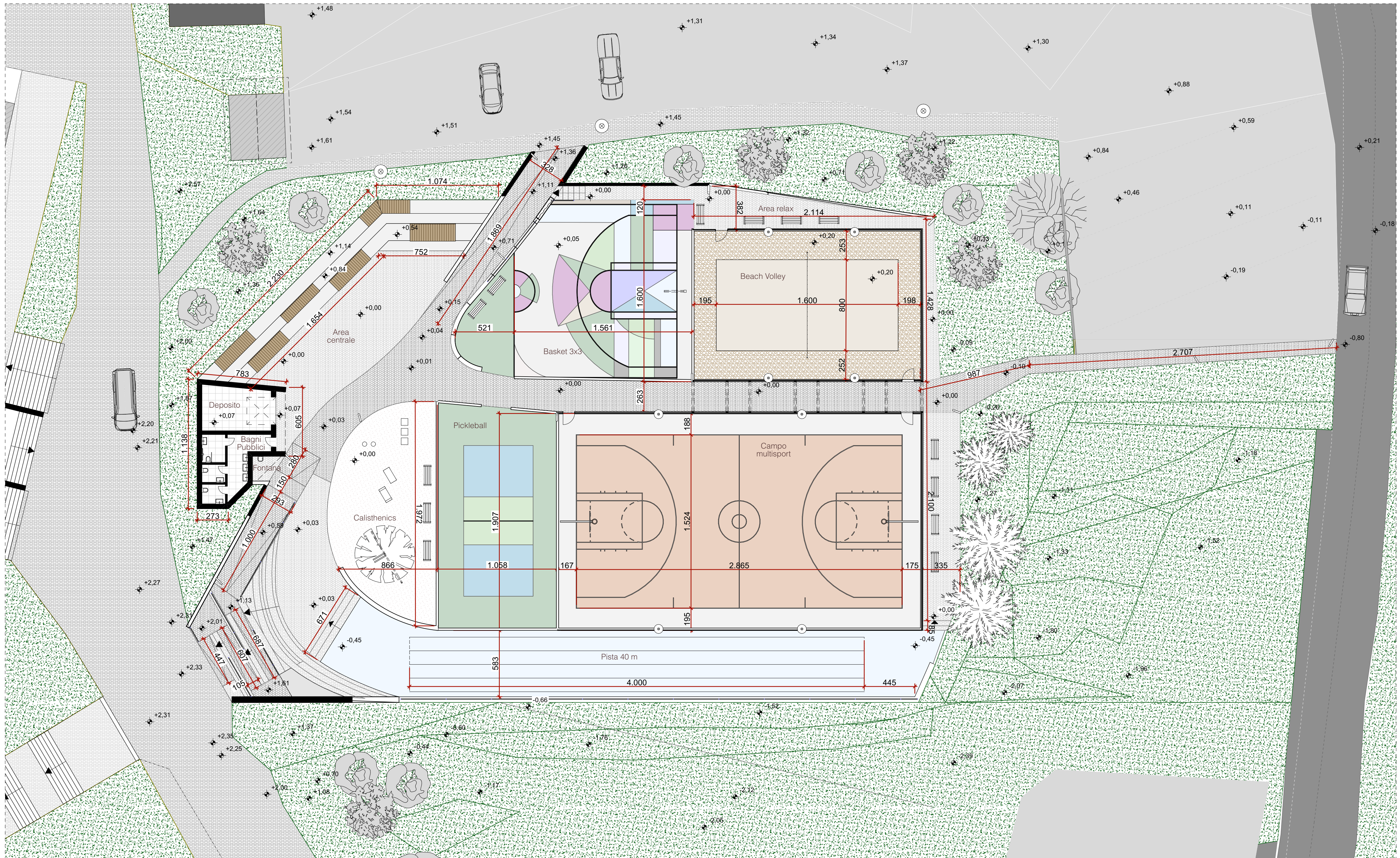
PLANIMETRIA PROGETTO - SCALA 1:200
